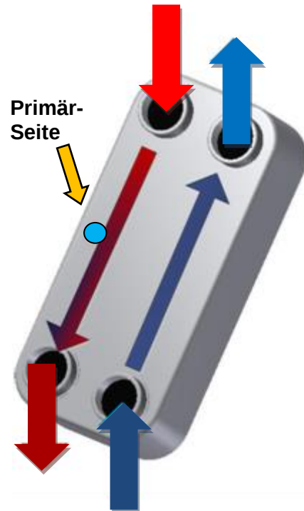
Abbildung 2: Allg. empfohlene Strömungsrichtung bei Plattenwärmeübertragern, sowie die Kennzeichnung der Primärseite
